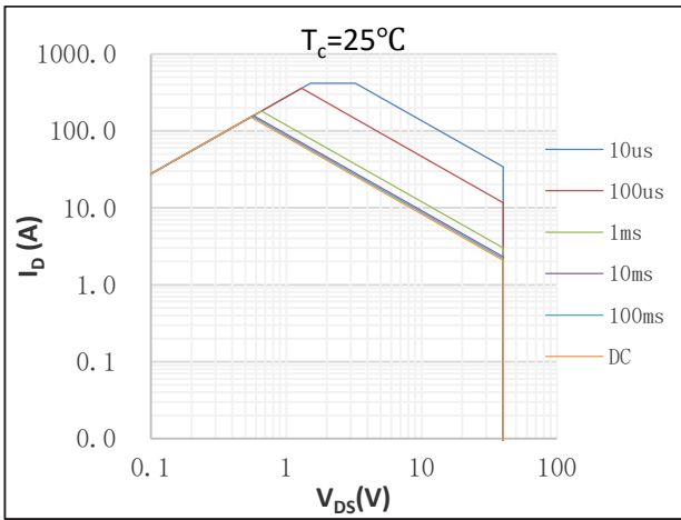
Fig.13 SOA
